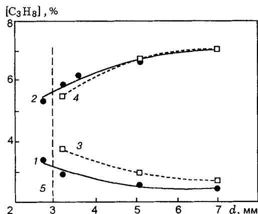
Рис. 2. Зависимость бедного (1) и богатого (2) концентрационных пределов распространения пламени в режиме НС от внутреннего диаметра трубки для смесей пропан — воздух: 3, 4 — концентрационные пределы распространения в трубке в режиме проскока, 5 — критический диаметр
