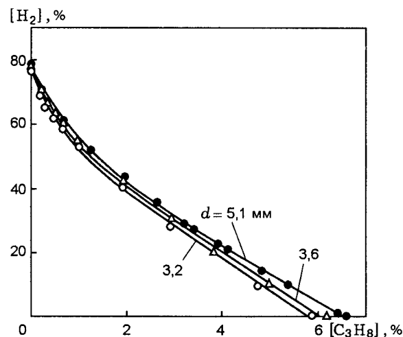
Рис. 4. Зависимость богатого концентрационного предела распространения пламени в режиме НС в смесях водород — воздух от концентрации пропана
