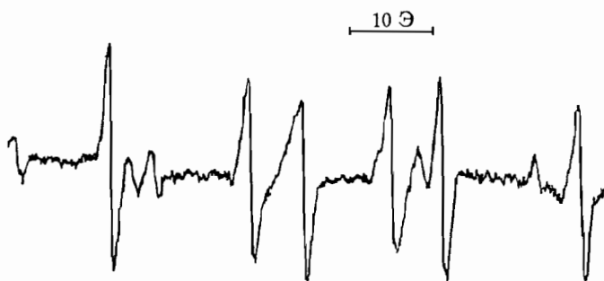
Спектр ЭПР спинового аддукта ловушки ГДПО при фотолизе паров триэтиламина
