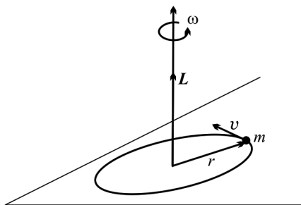
Рис. 1.1. Иллюстрация понятия «момент количества движения»
