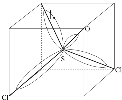
Рис. 6.4. Геометрическая структура молекулы \text{SOCl}_2
