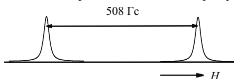
Рис. 7.17. Спектр ЭПР атомов водорода
