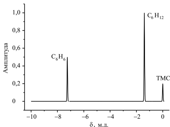
Рис. 7.23. Спектры ПМР циклогексана и бензола
