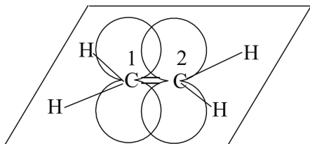
Рис. 5.25. \pi -система этилена
