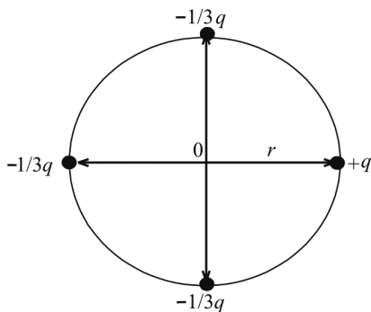
Рис. 5.29. Расположение обсуждаемой системы зарядов на плоскости
