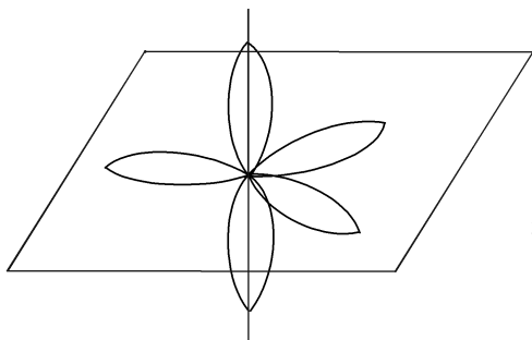
Рис. 6.1. Расположение пяти эквивалентных электронных пар вокруг центрального атома: электронные облака направлены к вершинам тригональной бипирамиды
