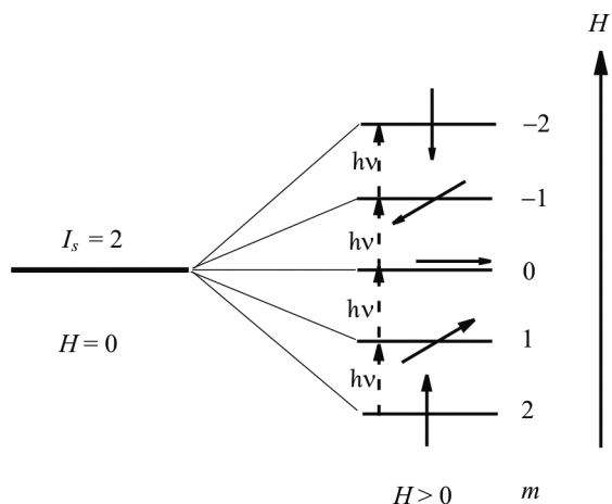
Рис. 7.20. Магнитный резонанс в случае четырех эквивалентных протонов
