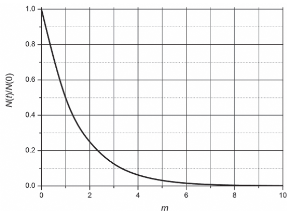
Рис.1.2. Зависимость N(t)/N(0) от t для случайного самопроизвольного распада
