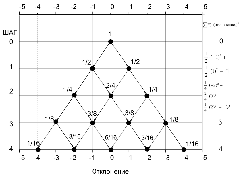
Рис. 8.8. Иллюстрация диффузионного движения.
