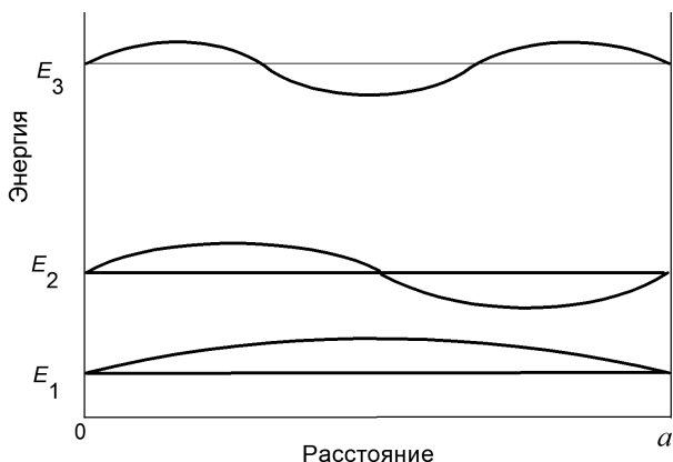
Рис. 2.6. Волновые функции и уровни энергии, описывающие стационарное движение микрочастицы в прямоугольной яме с бесконечно высокими стенками
