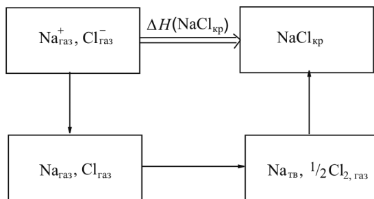
Рис. 11.2. Цикл Борна — Хабера
