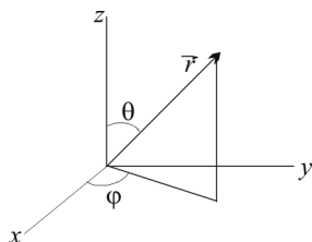
Рис. 3.2. Сферическая система координат
