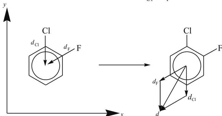
Рис. 5.31. Структура дипольного момента плоской молекулы орто -хлорфторбензола
