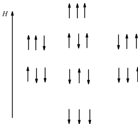
Рис. 7.19. Возможные ориентации ядерных спинов атомов водорода в радикале \cdot\text{CH}_3 , находящемся во внешнем магнитном поле H
