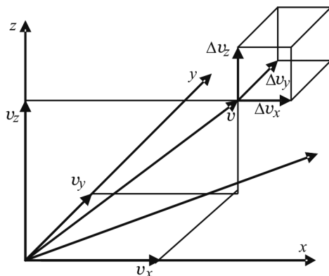
Рис. 8.1. Разложение скорости молекулы на составляющие
