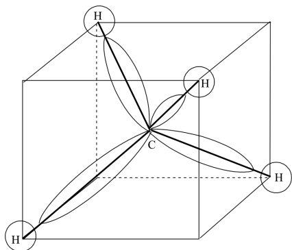
Рис. 5.12. Гибридизация типа sp^3
