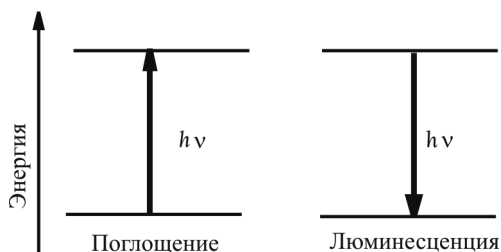
Рис. 7.2. Схема поглощения квантов света и люминесценции
