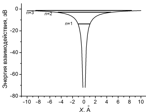
Рис. 3.1. Уровни энергии в атоме водорода
