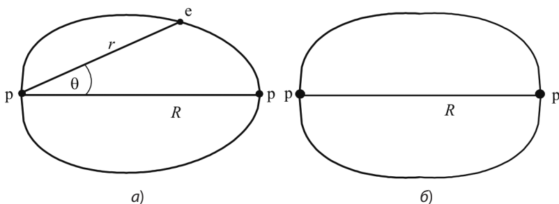
Рис. 5.3. Область связывания в плоскости трех частиц, p — протон, e — электрон:
