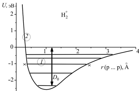
Рис.17.4. Мономолекулярный распад молекулы \text{H}_2^+
