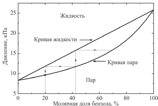
Рис. 14.3. Фазовая диаграмма «давление – состав» для системы «толуол – бензол» при температуре 41°C Показано также разделение перегонкой жидкой смеси, содержащей исходно 20 мол. % бензола
