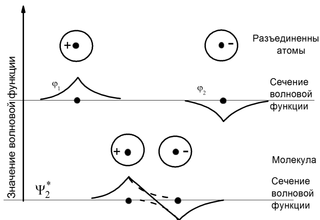
Рис. 5.15. Образование разрыхляющей орбитали молекулы водорода
