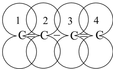
Рис. 5.26. \pi -система бутадиена
