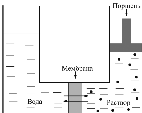
Рис. 14.6. Схема устройства для наблюдения осмотического давления
