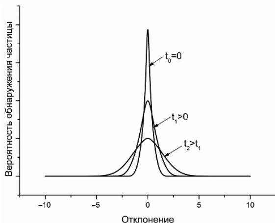
Рис. 8.9. Изменение вероятности обнаружения частицы со временем
