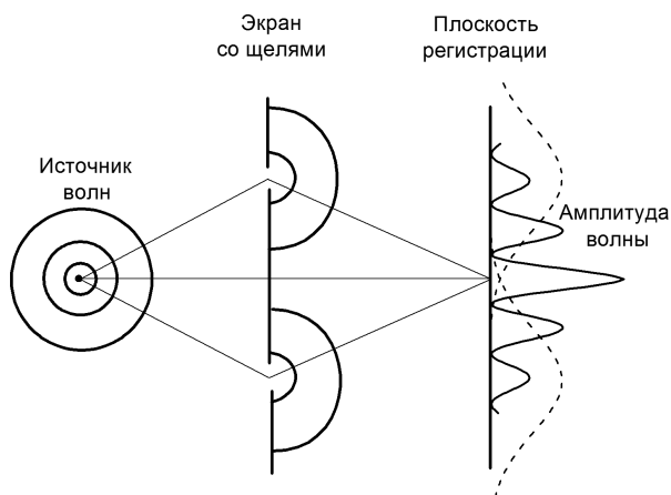
Рис. 2.4. Прохождение волны через две щели
