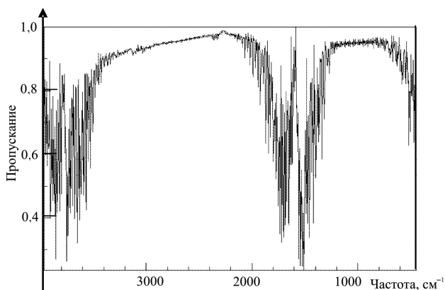
Рис. 7.9. Спектр ИК-поглощения молекул воды в газовой фазе
