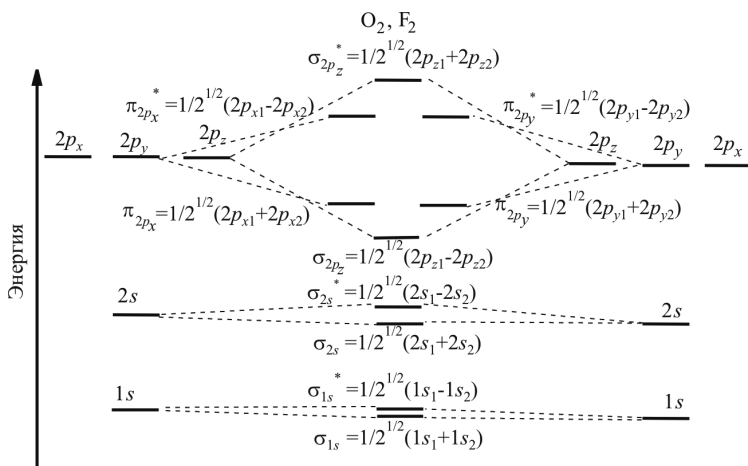
Рис. 5.18. МО гомоядерных молекул с участием кислорода и фтора
