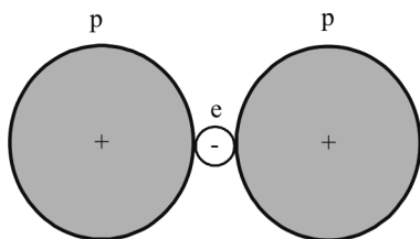
Рис. 5.5. Структура молекулы \text{H}_2^+ в предположении классического характера движения электрона и ядер. Обозначения: p — протоны, e — электрон
