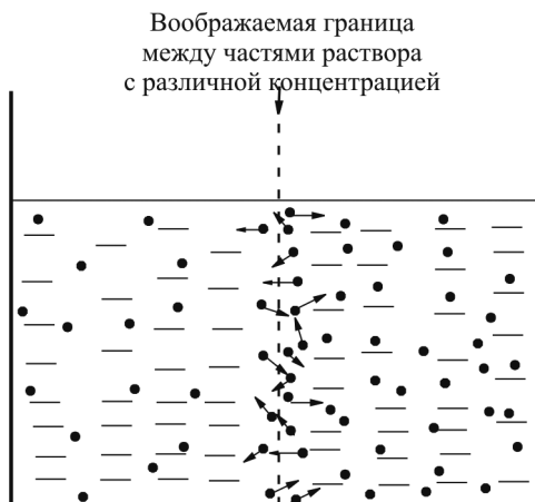
Рис. 8.7. Процесс перемешивания раствора за счет диффузии Точки — молекулы растворенного вещества. В правой части раствора концентрация выше в два раза. Видно, что вблизи воображаемой границы молекулы справа переходят в левую часть раствора в два раза чаще, чем при переходе слева направо
