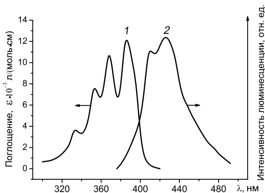
Рис. 7.6. Электронный спектр поглощения (1) и спектр люминесценции (2) 9,10-дифенилантрацена
