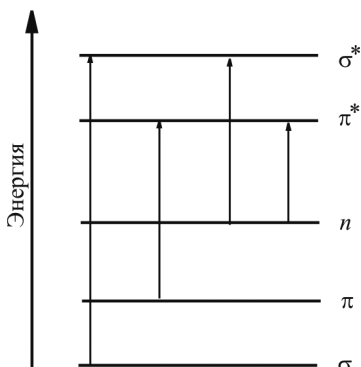
Рис. 7.4. Схема электронных переходов между уровнями, которым соответствуют указанные типы МО
