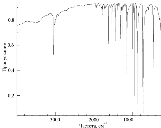
Рис. 7.10. ИК-спектр поглощения антрацена в растворе \text{CCl}_4
