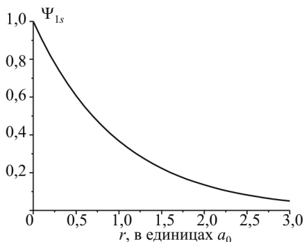
Рис. 3.3. Зависимость \Psi_{1s} от расстояния. Значения функции нормированы на ее величину в при r = 0
