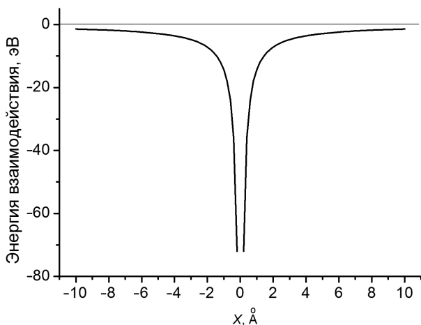
Рис. 2.5. Энергия взаимодействия электрона и протона
