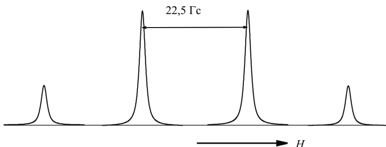
Рис. 7.18. Спектр ЭПР радикала \bullet\text{CH}_3
