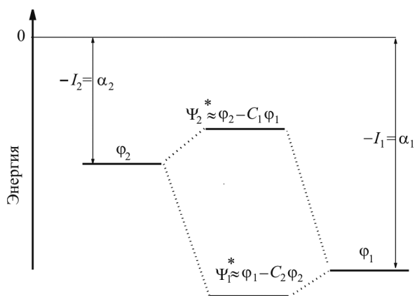
Рис. 5.19. Взаимодействие нерезонансных уровней энергии
