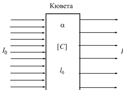
Рис. 7.3. Прохождение света через кювету с веществом
