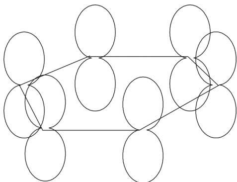
Рис. 7.22. \pi -Система молекулы бензола
