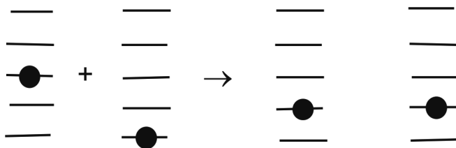
Рис. 9.3. Процесс передачи энергии от одного осциллятора к другому. Левый осциллятор возбужден на второй колебательный уровень энергии. В результате взаимодействия с невозбужденным осциллятором, один квант колебательной энергии переходит от возбужденного осциллятора к невозбужденному, и оба осциллятора оказываются возбужденными на первый колебательный уровень энергии
