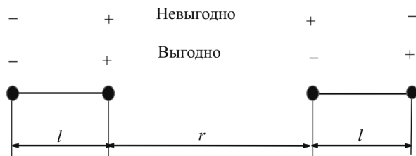
Рис. 8.4. Схема взаимодействия двух электрических диполей при их энергетически самой выгодной и самой невыгодной ориентациях
