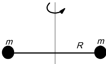
Рис. 2.9. Модель простейшего ротатора
