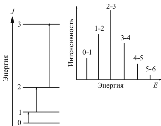
Рис. 7.11. Схема вращательного спектра
