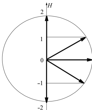
Рис. 7.14. Проекция спина l = 2 на ось магнитного поля
