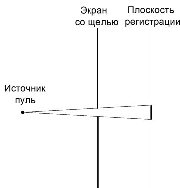
Рис. 2.3. Прохождение пуль через щель
