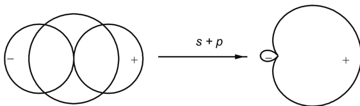
Рис. 5.9. Образование гибридных орбиталей при сложении s - и p -орбиталей
