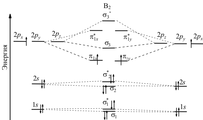
Рис. 5.22. Электронная структура молекулы бора B_2
