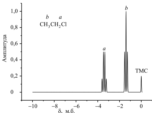
Рис. 7.24. Спектр ПМР хлористого этила
