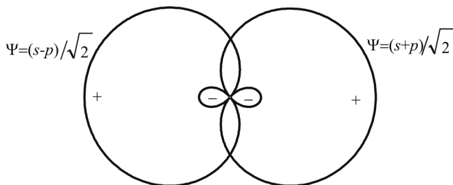
Рис. 5.10. Гибридизация типа sp
