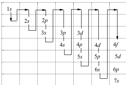
Рис. 4.2. Графическая иллюстрация правила заполнения электронных оболочек атомов
