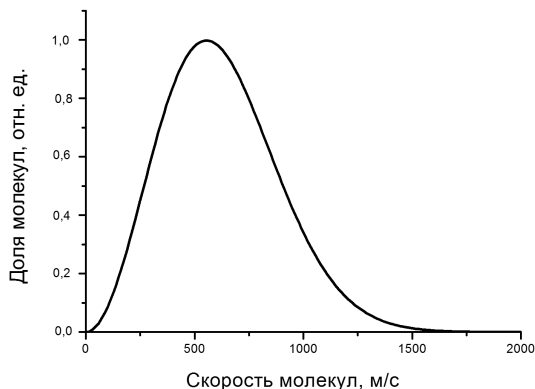
Рис. 8.3. Распределение Максвелла для молекул метана при 298,15 К, задаваемое формулой (8.6)
