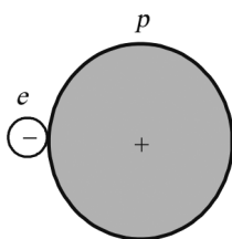
Рис. 3.11. Вид атома Н в предположении классического характера движения электрона и ядра ( p — протон, e — электрон)
