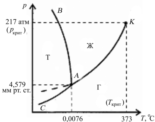
Рис. 13.1. Фазовая диаграмма воды
