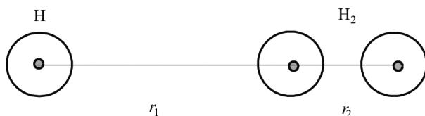
Рис. 17.1. Сближение атома водорода и молекулы водорода
