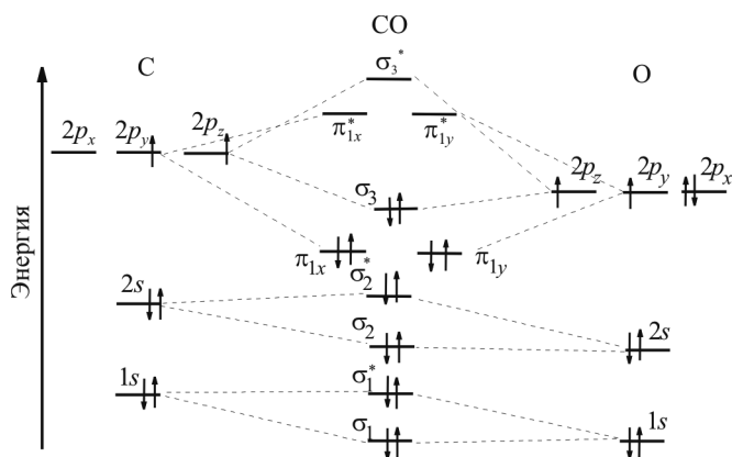
Рис. 5.24. Электронная структура молекулы СО
