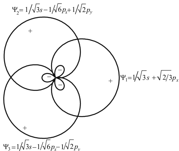
Рис. 5.11. Гибридизация типа sp^2
