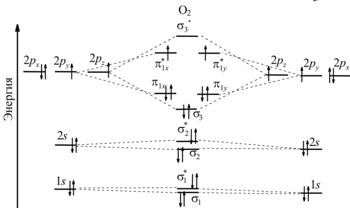
Рис. 5.23. Электронная структура молекулы O_2
