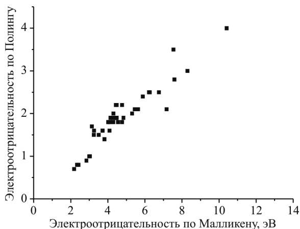
Рис. 5.28. Сопоставление электроотрицательностей по Полингу и Малликену
