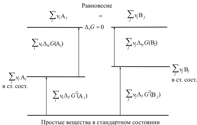
Рис. 12.1. Диаграмма изменения функции Гиббса в химическом равновесии (ст. сост. — стандартное состояние)
