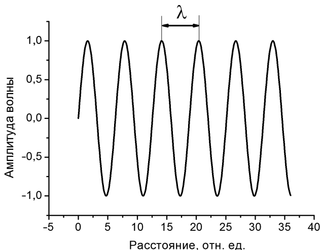
Рис. 2.1. Поведение волны в пространстве
