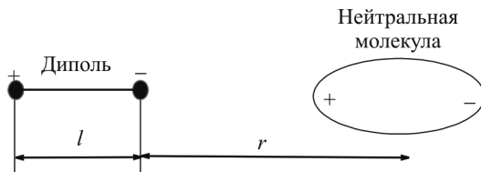
Рис. 8.5. Схема взаимодействия электрический диполь — нейтральная молекула
