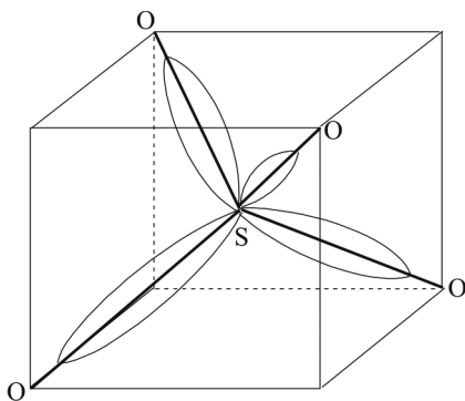
Рис. 6.3. Геометрическая структура молекулы SO_4^{2-}
