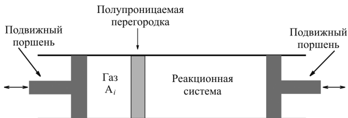
Рис. 12.2. Введение газа A_i в реакционную систему с сохранением парциального давления
