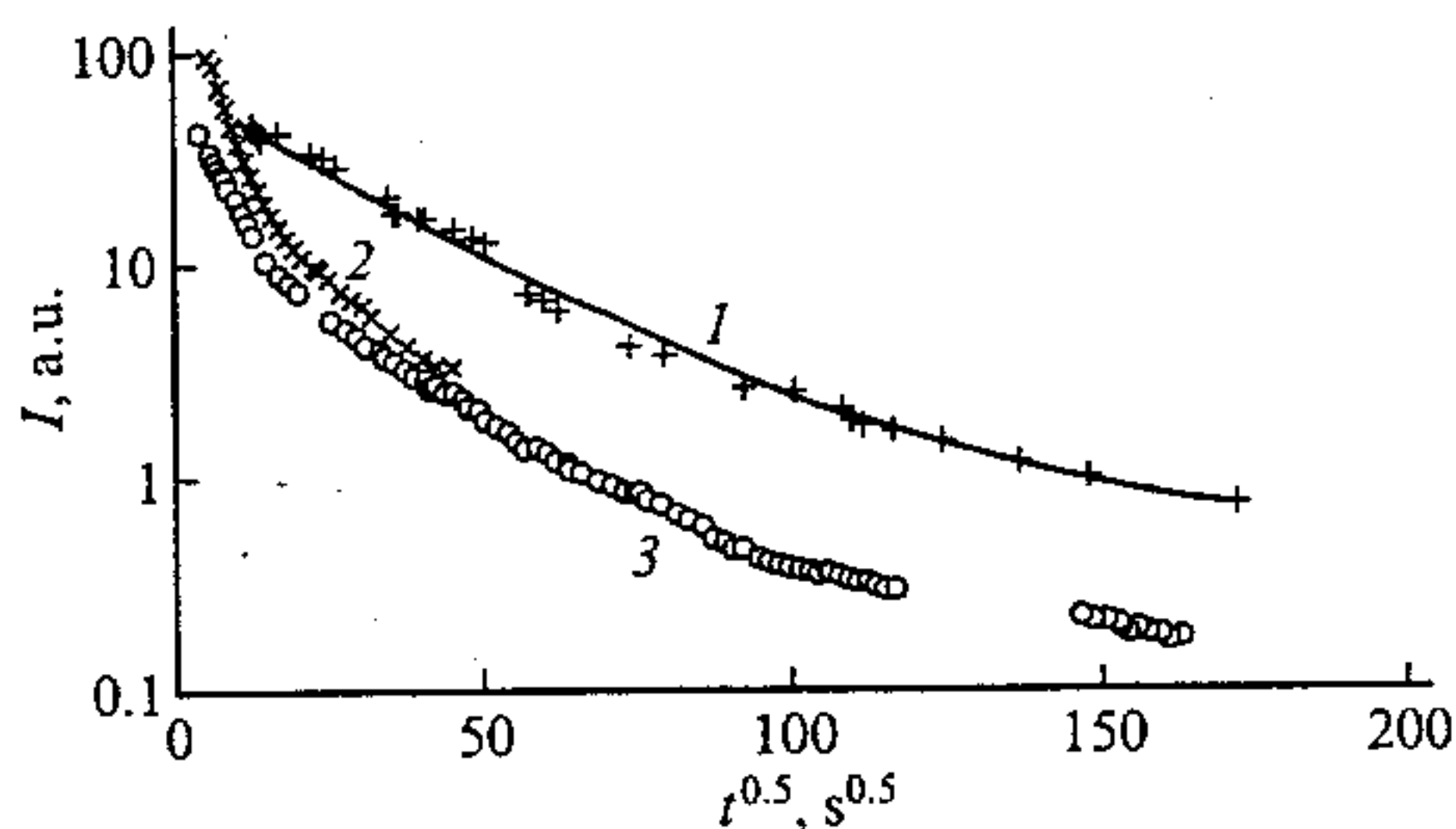
Рис. 1. Релаксация тока K^+ с нагретой проволоки: 1 — W при 1530 K, 2 — W при 1760 K, 3 — Pt при 1490 K.
