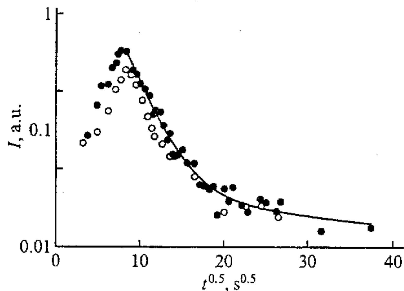
Рис. 3. Релаксация тока K^+ с W проволоки на ее охлаждение: — от 2300 до 1830 К, о — от 2140 до 1830 К. Кривая — аппроксимация.
