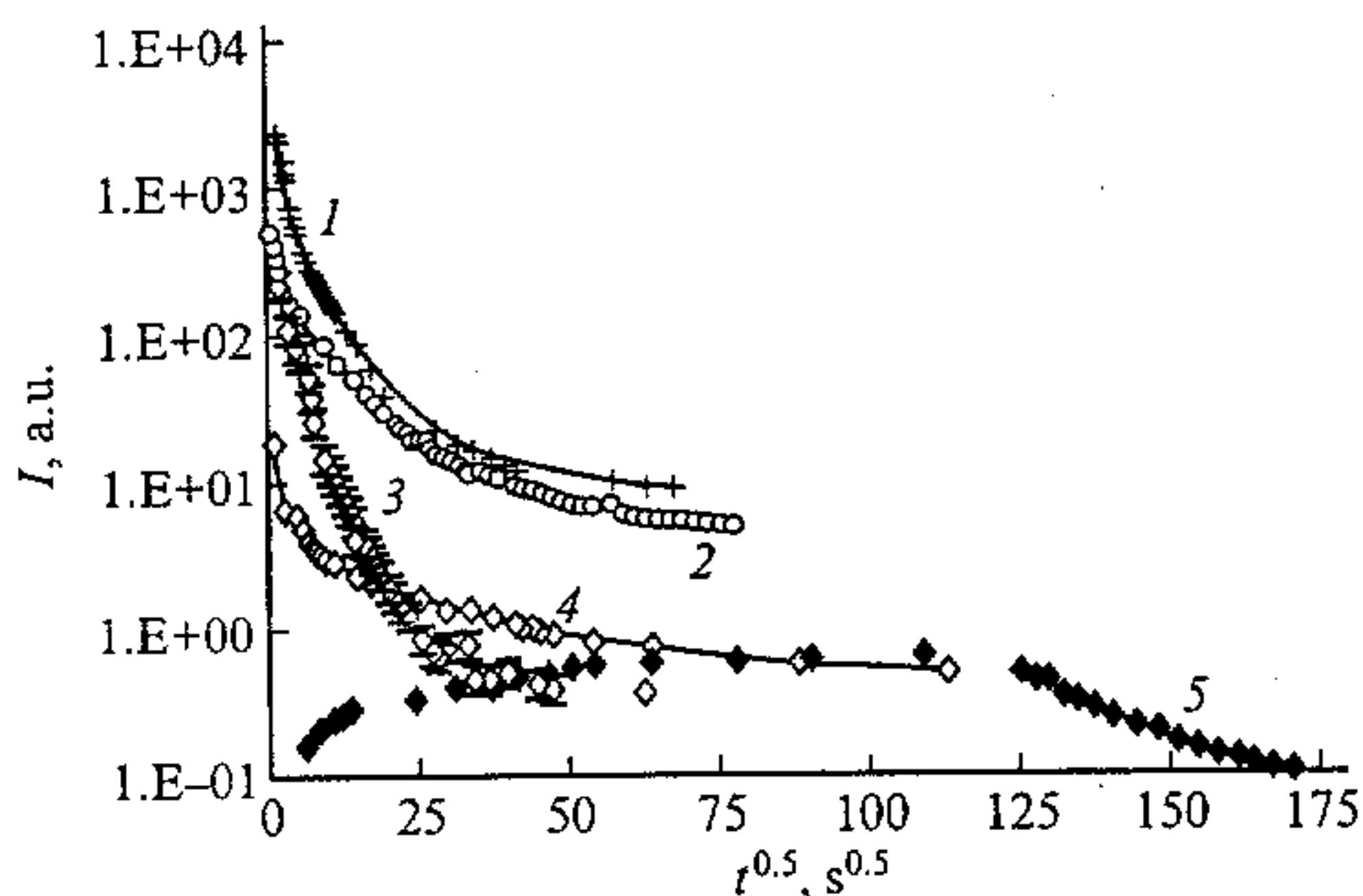
Рис. 2. Релаксация тока K^+ с нагретой проволоки после отжига в вакууме и контакта с H_2O : 1 — нихром при 1000 K, 2 — Pt при 1400 K, 3 — Mo при 1400 K, 4 и 5 — W при 1650 и 850 K.
