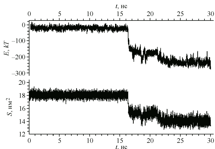
Рис. 2. Установление момента возникновения димера ГК в одной из прогонок модели с двумя молекулами ГК. Сверху — энергия леннард-джонсовского взаимодействия E_{LJ} , см. текст. Внизу для той же модели — суммарная площадь поверхности доступной для растворителя (для обеих молекул ГК). Кривые испытывают скачок примерно на 16 нс, который указывает, что молекулы встретились. Дополнительный скачок при 21 нс означает, что установился более оптимальный контакт молекул
