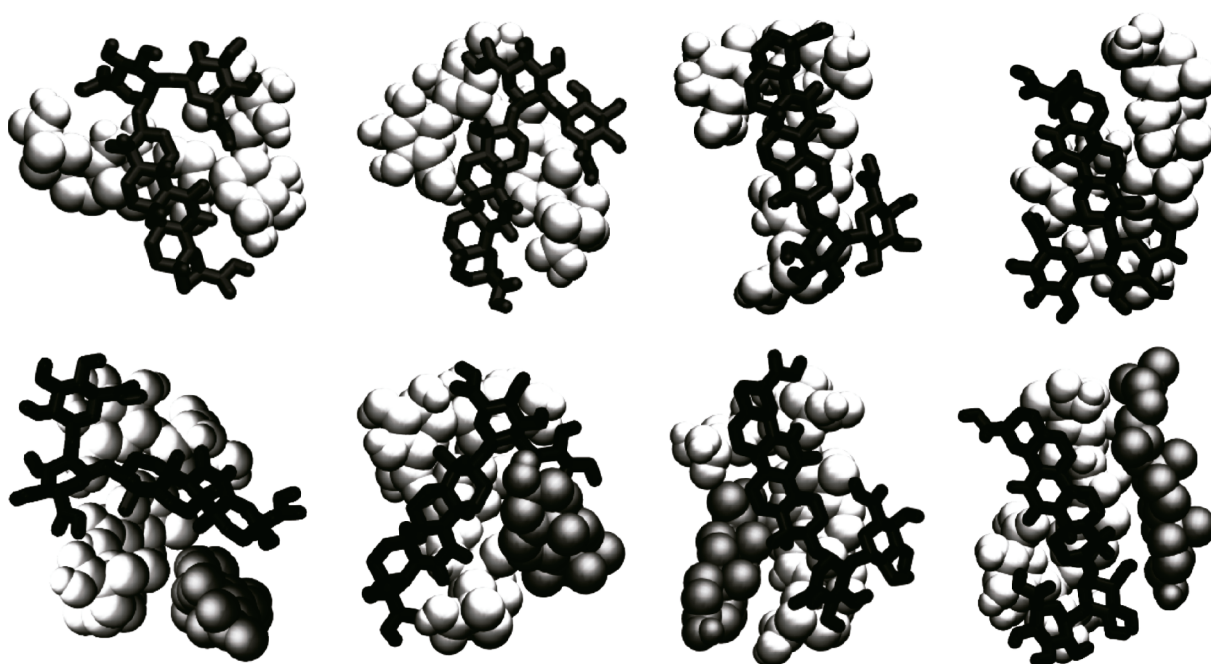
Рис. 8. Димеры ГК, соответствующие пятнам 1—4, на рис. 7 (а). Для ясности, одна из молекул ГК показана ван-дер-ваальсовыми атомами (светно-серые), а другая скелетом (а). Кластеры 2:1 из соответствующих пятен на рис. 7 (б). Молекула холестерина показана темно-серым
